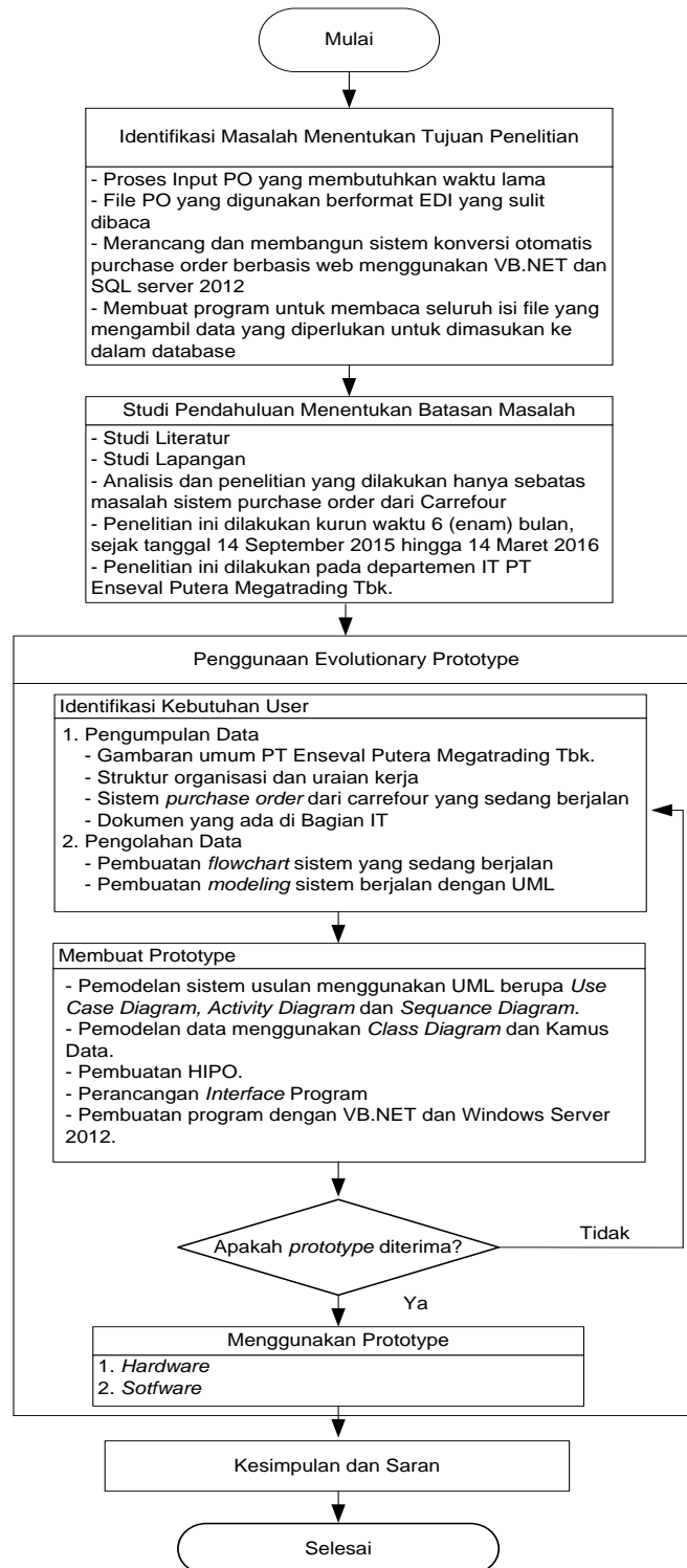
Gambar III.1 Kerangka Penelitian (Sumber: Hasil Pengolahan Data, 2017)
