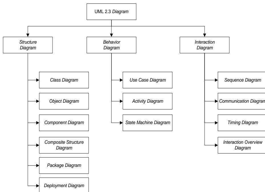
Gambar II.6 Klasifikasi Diagram UML (Sumber: Rosa dan Shalahuddin,2013)
